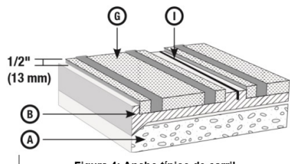
Figura 4: Ancho típico de carril sección de junta de expansión
