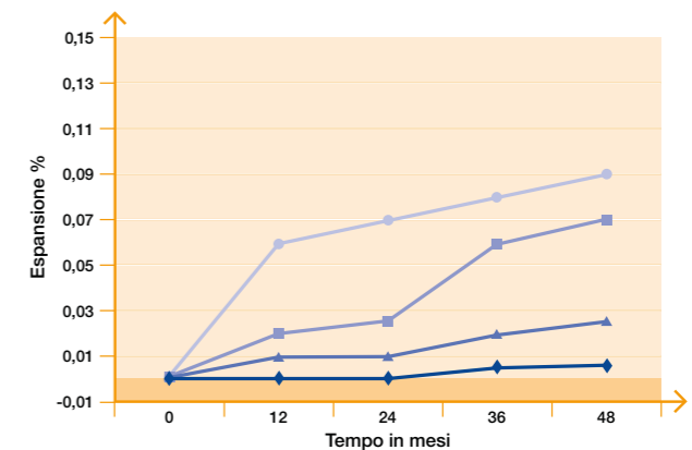
Effetto dell'aggiunta di MasterLife MS 610 su calcestruzzo confezionato con aggregati contenenti silice attiva
