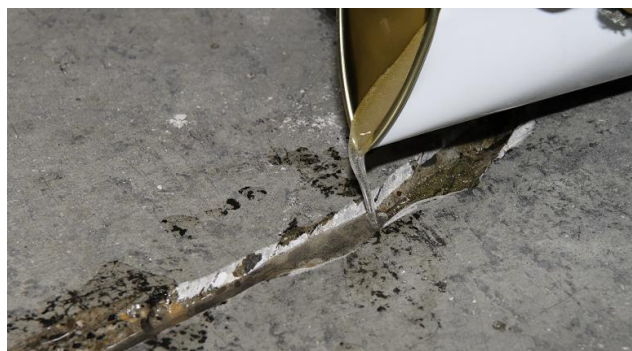
Rys. 4. Wylewanie MasterInject 1360 bezpośrednio w otwartą bruzdę w kształcie litery V w pęknięciu.
