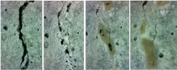
Pęknięcie
