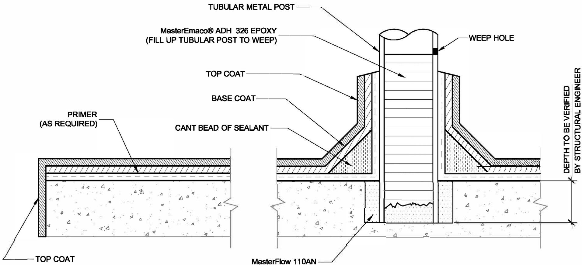
BALCONY EDGE - DC-13 N.T.S.
