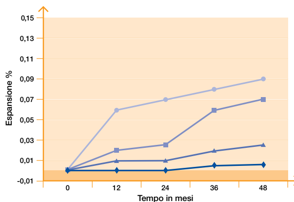
Effetto dell'aggiunta di MasterRoc MS 610 su calcestruzzo confezionato con aggregati contenenti silice attiva
